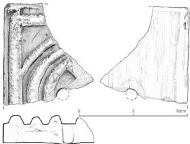
Obr. 4: Klášter, bývalý cisterciácký klášter Nepomuk. Zlomek obkladové terakotové desky. Zřetelný je otvor pro hřeb (kresba S. Svatošová, 2014).
