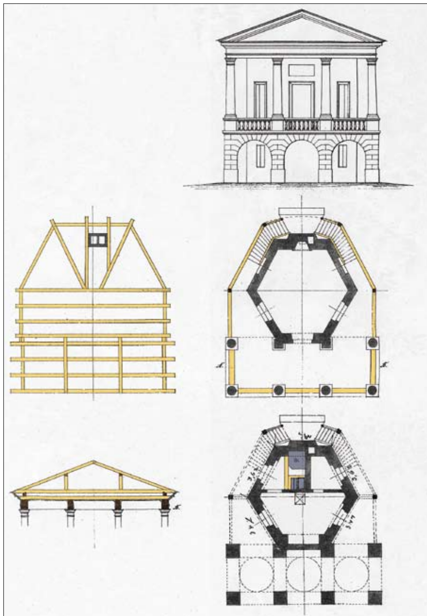
Obr. 3: Lednice, Lovecký zámek, plán na výměnu krovu a drobné úpravy v interiéru, J. Ohnsorg, nedat. (repro, originál Moravský zemský archiv v Brně, fond F 115 Liechtensteinský stavební úřad Lednice, č. 4389).
