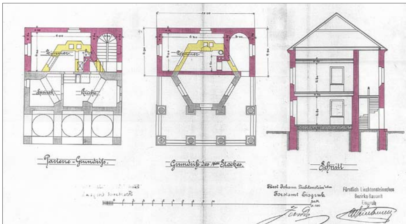
Obr. 6: Lednice, Lovecký zámek, plán přestavby, K. Weinbrenner, 1900 (repro, originál Státní oblastní archiv Břeclav se sídlem v Mikulově, fond B 35 Archiv městečka Lednice, č. 270).
