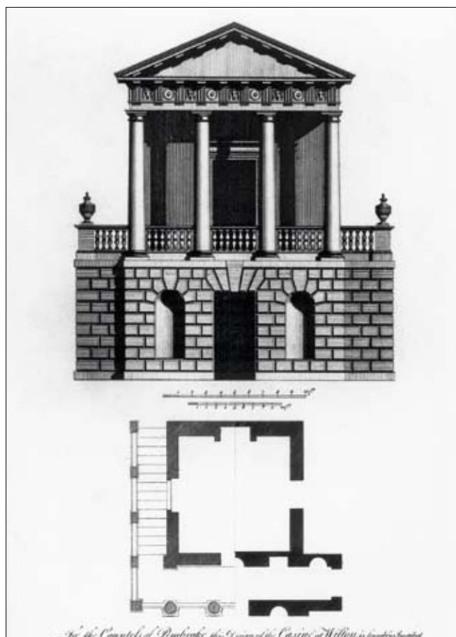
Obr. 7: W. Chambers, Casino hraběte Pembroka ve Wiltonu 1791 (repro z W. Chambers, A Treatise on the Decorative Part of Civil Architecture . London 1791, s. 37 (3. vydání; 1. vydání 1759).
