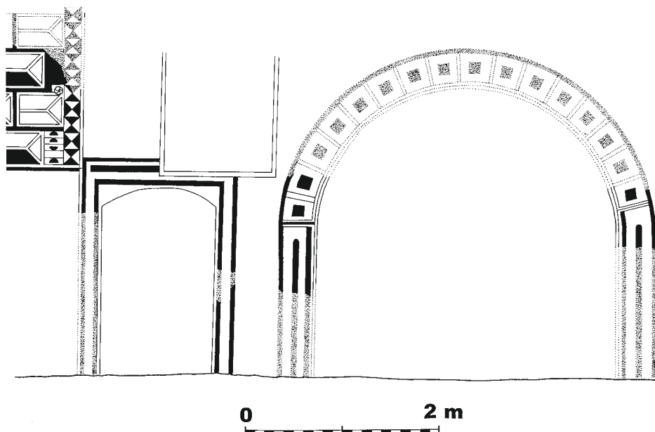
Obr. 12: Lustenec, dvůr. Sgrafitová výzdoba původní vjezdové brány a branky na jihozápadní straně (dnes zazděno). Zaniklé a pod omítkou skryté části výzdoby doplněny tečkovaně, viditelné vyznačeny černě (zaměření a kresba D. Kovář, 2004).
