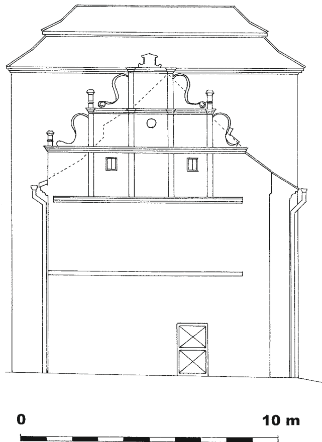
Obr. 17: Předměstí Českých Budějovic, Pillmannův (Ehrenpreisův) dvůr. Východní průčelí obytné budovy s renesančním štítem. Nad ním ční nástavba ve střední části budovy (kresba D. Kovář, 2005).
