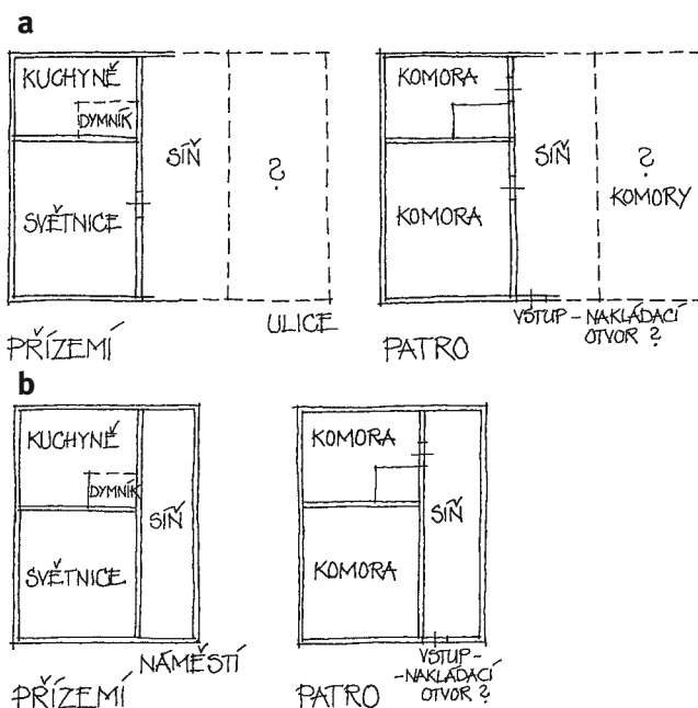
Obr. 19: Bělá pod Bezdězem, schéma původních dispozic domů ze 17. století; a – dům čp. 4, b – dům čp. 18 (kresba E. Vyletové).
