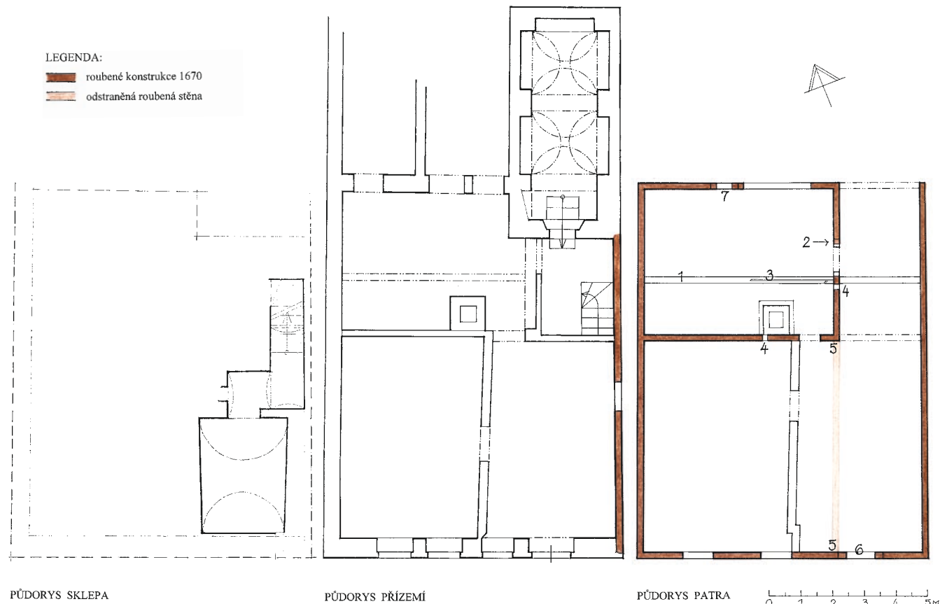
Obr. 13: Bělá pod Bezdězem, dům čp. 18, zaměření domu, půdorys přízemí, patra a sklepa, (zaměření a kresba E. Vyletová 2010; zaměření sklepa převzato z projektu stavebních úprav, P. Řezáč, 2008). 1 – původní stropní trám, 2 – kapsa po původním stropním trámu, 3 – žlábek v horní ploše stropního trámu nad přízemím viditelný po rozkrytí podlahy, 4 – otvor po vodorovném trámu konstrukce dymníku, 5 – odřezaná zhlaví roubené stěny, 6 – okno s dochovanými stojkami původního vstupu, 7 – okno do dvora s původními stojkami.
