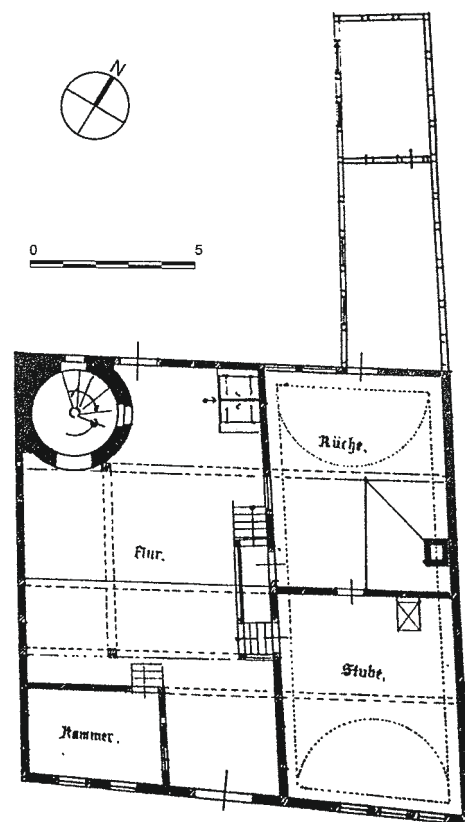
Obr. 21: Schmalkalden, Německo, dům čp. 25, Stumpfengasse, půdorys přízemí (převzato z: P. Zalewski, o. c. v pozn. 27, s. 347). Příklad dispozice domu z doby kolem roku 1600, pro níž je charakteristické umístění vytápěné světnice („Stube“) s navazujícím prostorem kuchyně v přízemí. I když se v daném případě na rozdíl od bělských domů jedná o honosný měšťanský dům s rozlehlou síní, základní schéma půdorysu je obdobné.
