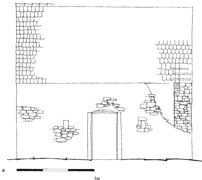
Obr. 12: Líšina, usedlost čp. 46. Sýpka při východní straně dvora: a – pohled (západní strana); b – půdorys (kresba K. Foudl).
