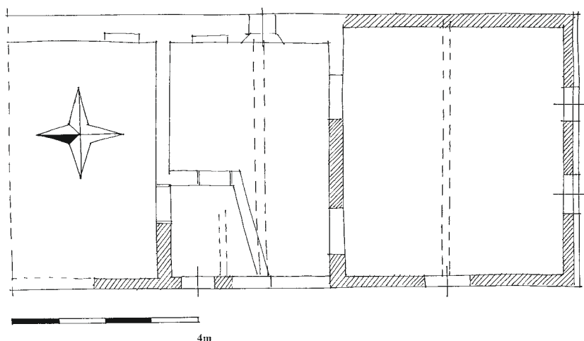
Obr. 3: Líšina, usedlost čp. 46. Půdorysné schéma obytného domu se světnicí v přední části, síní a někdejší černou kuchyní uprostřed a druhou světnicí (též komorou) v zadní části domu – zprava (kresba K. Foud, 2014).
