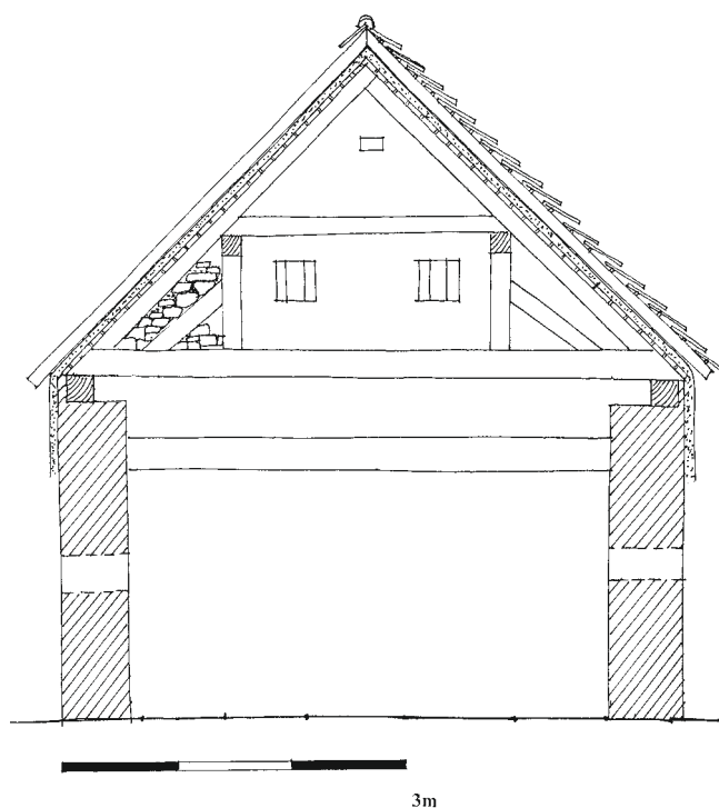
Obr. 13: Líšina, usedlost čp. 46, sýpka za obytným stavením. Řez, pohled na jižní/vnitřní stranu severní zdi (kresba K. Foudl).
