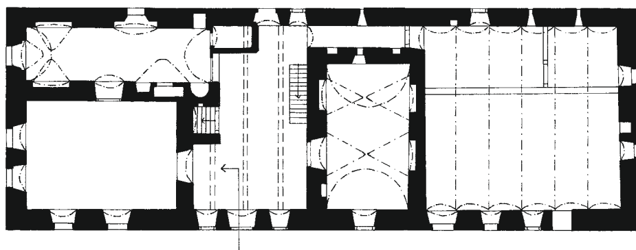
Obr. 27: Hrušová, čp. 10, zaměření přízemí a patra domu (zaměření Z. Vařeková a J. Švec, kresba J. Švec, 2014).
