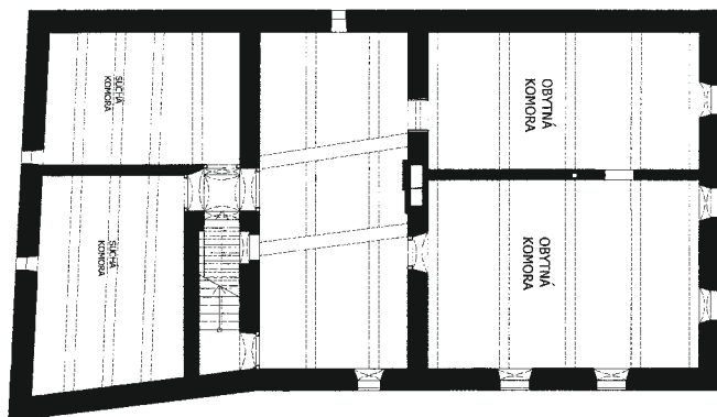
PŮDORYS 1. PATRA 1 : 100
