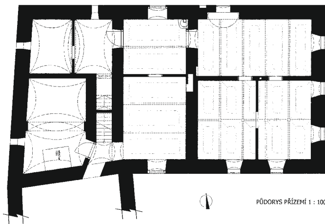
Obr. 32: Hrušová, čp. 30, zaměření přízemí a patra domu (zaměření poskytnuto majitelem usedlosti p. Kroulíkem, upravil J. Švec, 2014).
