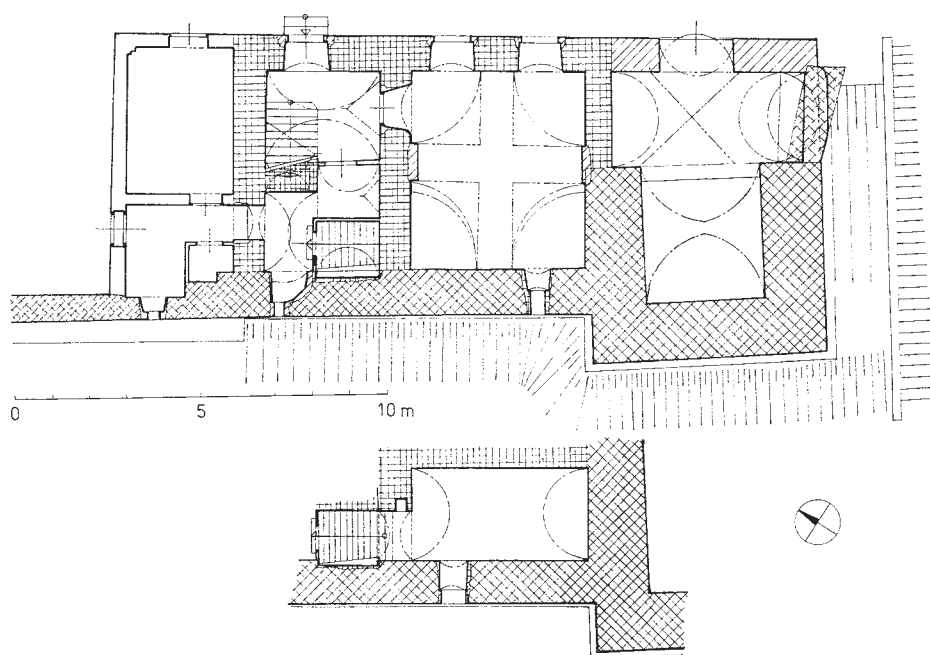
Obr. 3: Broumov, děkanství čp. 22 – půdorys přízemí a suterénu. Zdivo: mřížkovaně – gotické; mřížkovaně ke kolmo konstrukci – renesanční; šrafovaně – barokní (zaměření a vyhodnocení J. Čížek a J. Slavík, 1986–1988).
