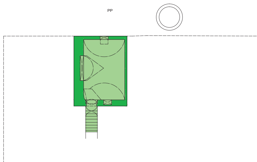
Obr. 32: Frýdštejn, usedlost čp. 21 – půdorys PP s vyhodnocením stavebního vývoje (zaměření M. Ouhrabka, T. Konvalinková, L. Sodomková; kresby L. Sodomková (obr. 32–36); všechna vyhodnocení stavebního vývoje autoři).
