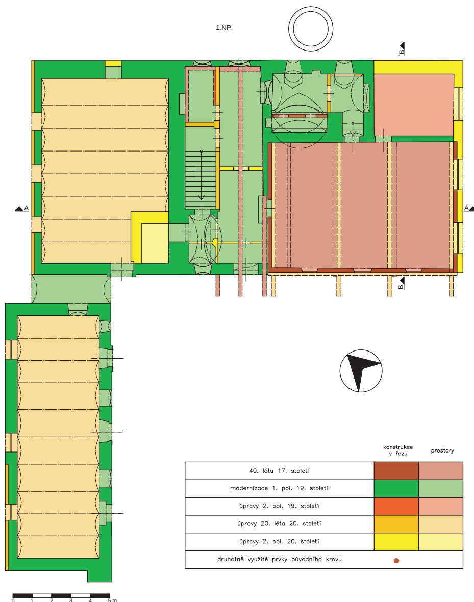
Obr. 33: Frýdštejn, usedlost čp. 21 – půdorys 1. NP s vyhodnocením stavebního vývoje (zaměření M. Ouhrabka, T. Konvalinková, L. Sodomková).
