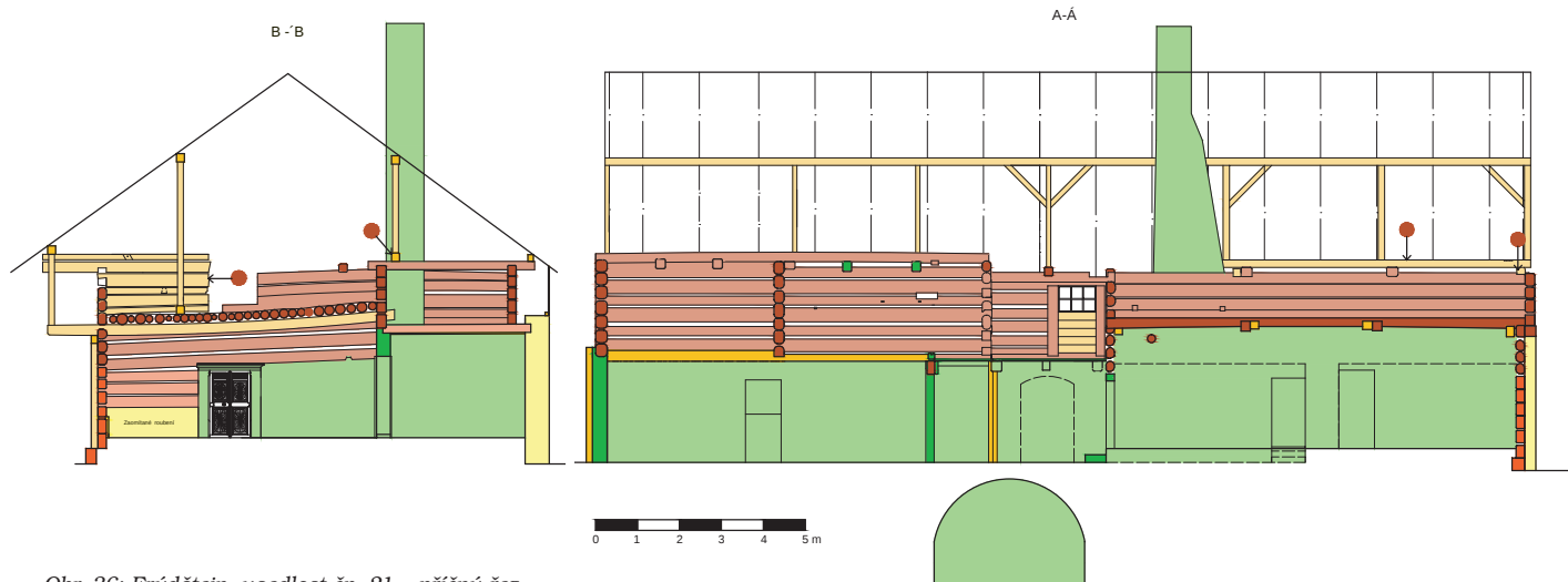
Obr. 36: Frýdštejn, usedlost čp. 21 – příčný řez s vyhodnocením stavebního vývoje (zaměření M. Ouhrabka, L. Sodomková).
