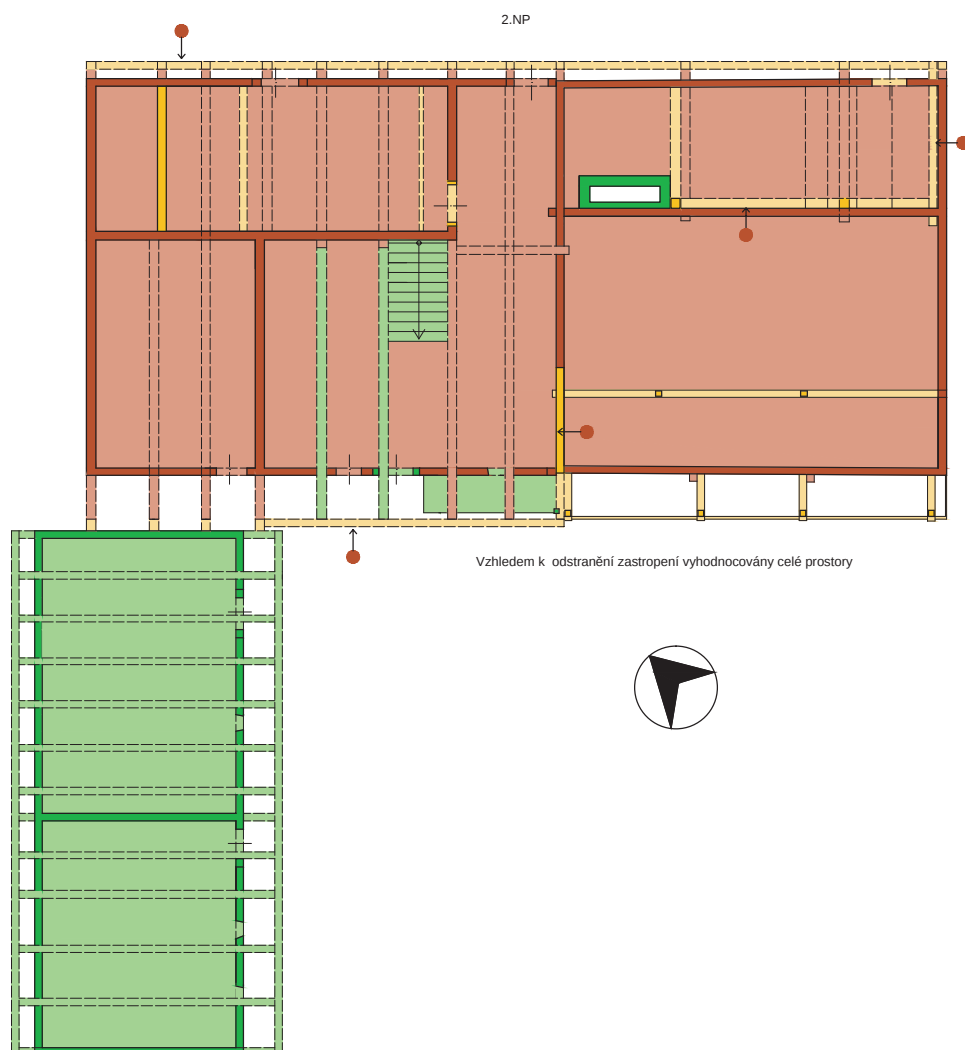
Obr. 34: Frýdštejn, usedlost čp. 21 – půdorys 2. NP s vyhodnocením stavebního vývoje (zaměření M. Kolka, I. Peřina, M. Ouhrabka, T. Konvalinková, L. Sodomková).
