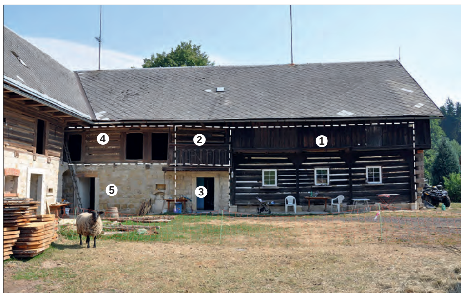
Obr. 11: Frýdštejn, usedlost čp. 21 – jihozápadní okapové průčelí s vyznačením historické dispozice: 1 – roubený blok obytného dílu s polopatrem; 2 – síň v patře; 3 – rozsah původní roubené síně v přízemí; 4 – komorové patro; 5 – prostor původně roubeného chléva (foto T. Konvalinková, srpen 2015).
