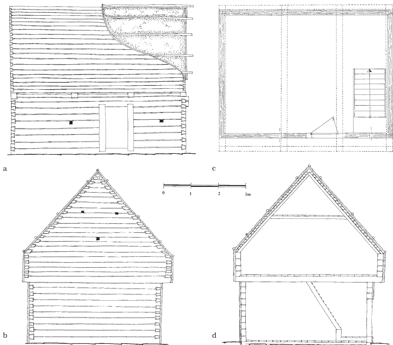
Obr. 15: Močerady, usedlost čp. 21, dnes Ohůčov. Sýpka z let 1819–1821. Pohled na původní jižní (nádvořní) a západní (štíťovou) stranu, půdorys přízemí a příčný řez.
