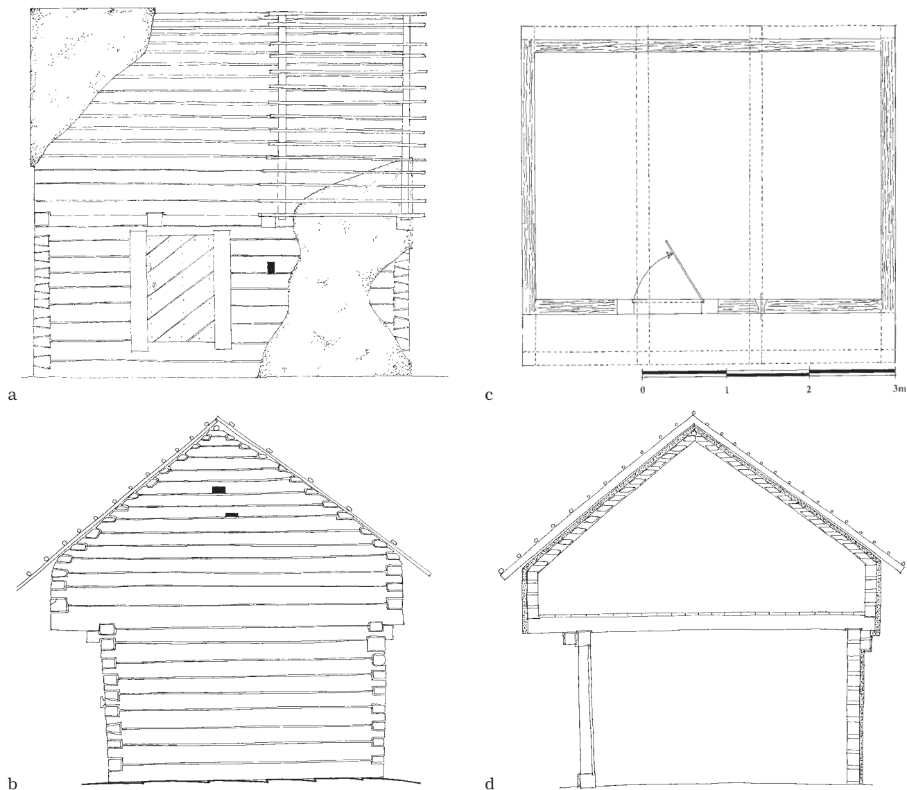
Obr. 12: Močerady, usedlost čp. 21, dnes Ohůčov. Sýpka z let 1781–1789. Pohled na: a – původní východní (nádvoří); b – severní (štítovou) stranu; c – půdorys přízemí; d – příčný řez.
