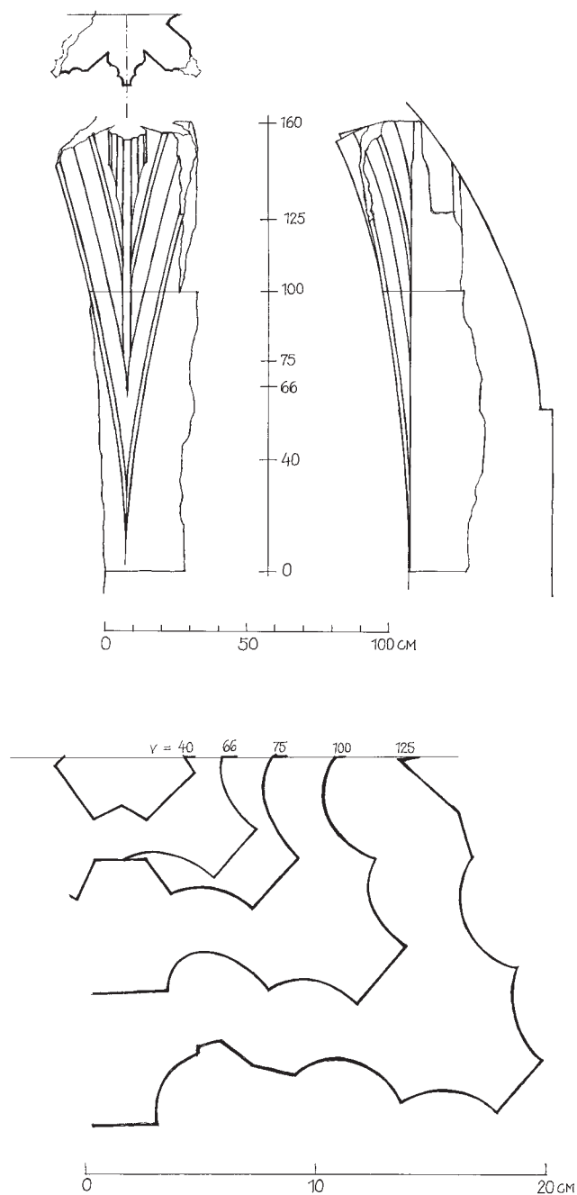
Obr. 3: Bělá pod Bezdězem, klášter: a – výběh žeber klenby, půdorys, čelní a boční pohled s vyznačením výškových kót měření profilace; b – profilace výběhu žeber, měřeno ve výšce 40, 66, 75, 100 a 125 cm nad patou výběhu, otisky snímány pomocí hřebenu. Snímání otisku profilace nad kótou 125 cm bylo problematické z důvodu narušení bočních žeber a špatné přístupnosti u navazující barokní zaddívky
