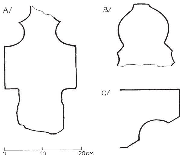
Obr. 6: Bělá pod Bezdězem, klášter – profilace architektonických článků odhalených při stavebních pracích v prostoru kaple a sakristie: a – fragment klenebního žebra s dvojitě vyžlabeným profilem; b – fragment klenebního žebra s hruškovým profilem; c – profilace čela pískovcové desky druhotně vsazené do konstrukce barokní menzy (profilace sejmuta pomocí hřebenu).
