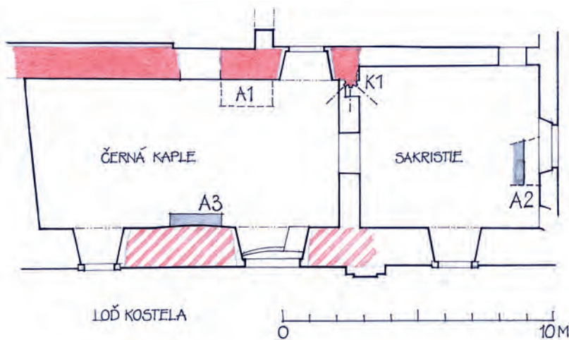
Obr. 2: Bělá pod Bezdězem, klášter – půdorys černé kaple a sakristie se zakreslením výběhu žebér klenby a nálezů z archeologického výzkumu (zaměření je orientační pro potřeby osvětlení situace nálezu). Červeně je vyznačeno zdivo gotického původu; červeně šrafované pravděpodobný gotický původ; K1 – výběh žebér; A1 – archeologická sonda, vlevo od sondy byly v severní stěně pod úrovní barokní podlahy viditelné svislé spáry se zazdívkou; A2 – v archeologické sondě byl ve vzdálenosti cca 0,6 metru od obvodové stěny zachycen líc pískovcového zdiva pravděpodobně gotického původu probíhající severojižním směrem; A3 – nález zdiva z pískovcových kvádrů; údaje poskytl J. Švédová, o. c. v pozn. 9 a 13; (všechna zaměření a kresby E. Vyletová, 2015).
