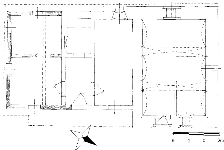
Obr. 23: Merklín – usedlost čp. 19. Půdorys obytného stavení. Schéma. Zleva přední světnice, uprostřed síň s navazující kuchyní (pův. černá kuchyně) a vpravo komora (též zadní světnice). Od severozápadu k obytné části přiléhaly zděné chlévy, vyzdvížené v průběhu druhé poloviny 19. století (kresba a zaměření K. Foud, 2014).
