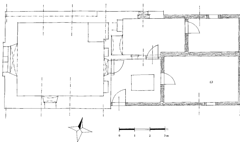
Obr. 16: Vlčice u Blovic – usedlost čp. 11. Půdorysné schéma obytného stavení. Zleva přední díl se světnicí, uprostřed střední díl se síní a blokem někdejší černé kuchyně a zadní díl se zadní světnicí a přilehlou komorou. Podélné šrafování značí roubené konstrukce. Světnice je kladena do roku 1832, zadní komora pochází z let 1767–1768 (zaměření a kresba A. Aubrechtová a K. Foud, 2013).
