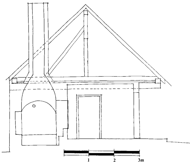
Obr. 7: Dolní Lukavice – stavení čp. 77/E5. Řez střední částí objektu (kresba K. Foud podle zaměření Ing. M. Kučerové, 2014)
