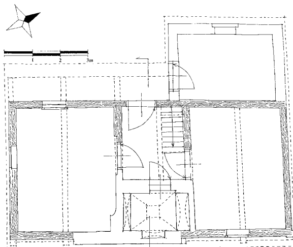
Obr. 8: Dolní Lukavice – stavení čp. 77/E5. Půdorys přízemí (kresba K. Foud podle zaměření Ing. M. Kučerové, 2014).
