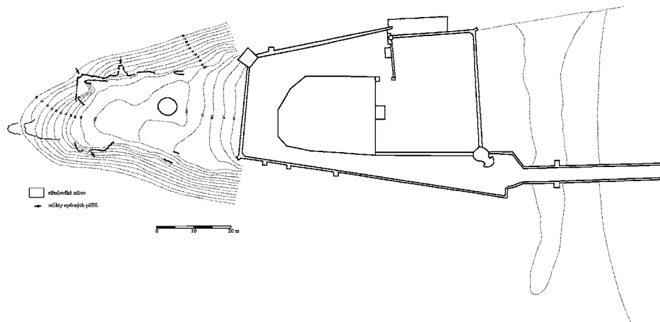
Obr. 1: Žaclěř (okres Trutnov), zámek čp. 1 - zaměření relikvů středověkého opevnění v jižní části hradního návrší, tzv. dolní hrad (zaměření I. Peřina, 2011). Jelikož se u horního hradu jedná o překreslenou situaci, která nebyla v rámci operativní dokumentace přeměřená, nejsou zde zakresleny vrstevnice (situace tzv. horního hradu převzata ze zaměření SÚRPMO, 1985).
