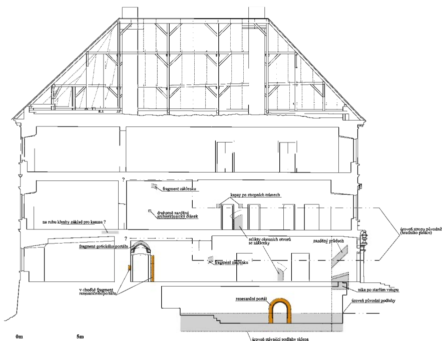
Obr. 5: Žacléř, zámek čp. 1 – podélný řez s vyznačením náleзовých situací (zákres M. Buroň).
