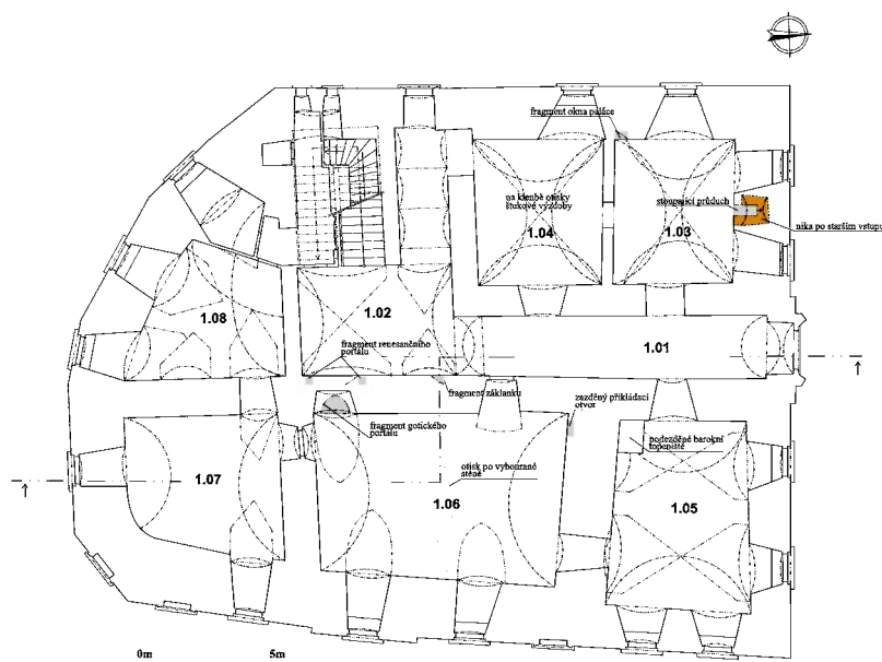
Obr. 2: Žacléř, zámek čp. 1 – půdorys přízemí s vyznačením nálezových situací (zákres M. Buroň).
