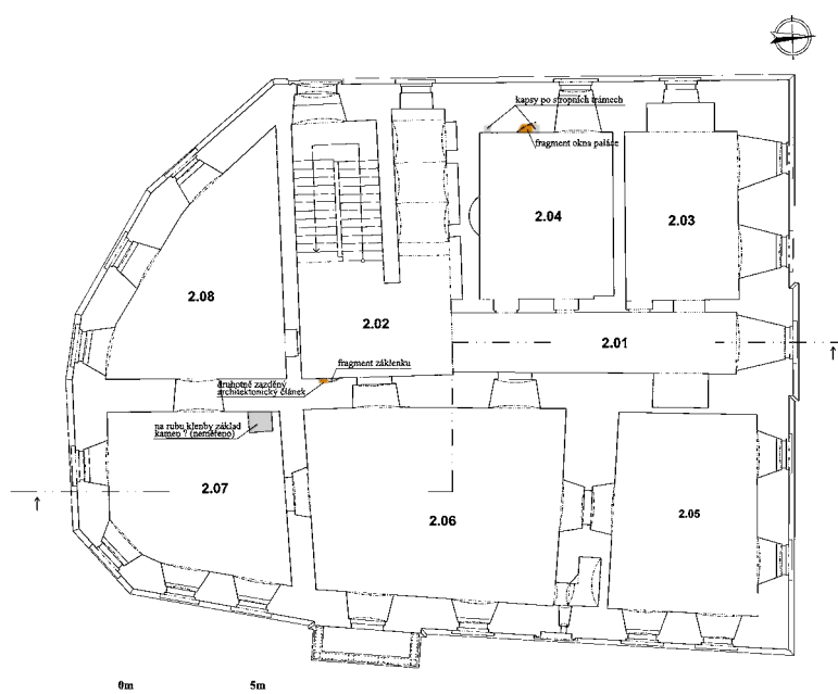
Obr. 4: Žacléř, zámek čp. 1 – půdorys 1. patra s vyznačením náleзовých situací (zákres M. Buroň).
