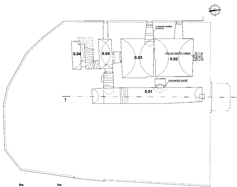
Obr. 3: Žacléř, zámek čp. 1 – půdorys sklepa s vyznačením nálezových situací (zákres M. Buroň).
