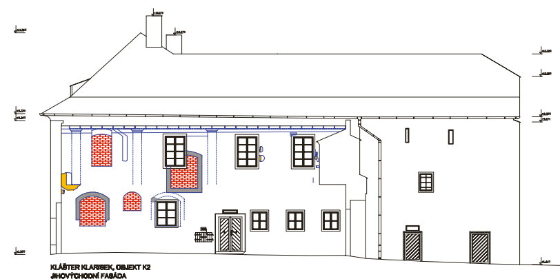
Obr. 56: Český Krumlov, Latrán čp. 67, hospodářský dvůr kláštera klarisek (zákres M. Špinarová).
