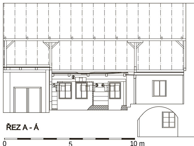
Obr. 26: Vyšší Brod, dům čp. 24, podélný řez domem (zaměření a zákres V. Babická).
