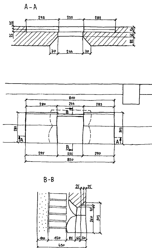
Obr. 21: Vyšší Brod, dům čp. 24, interiér roubené světnice, zákres horního větracího okénka s posuvnou okenicí a okosením na exteriérové straně (zaměření a zákres J. Eliška).
