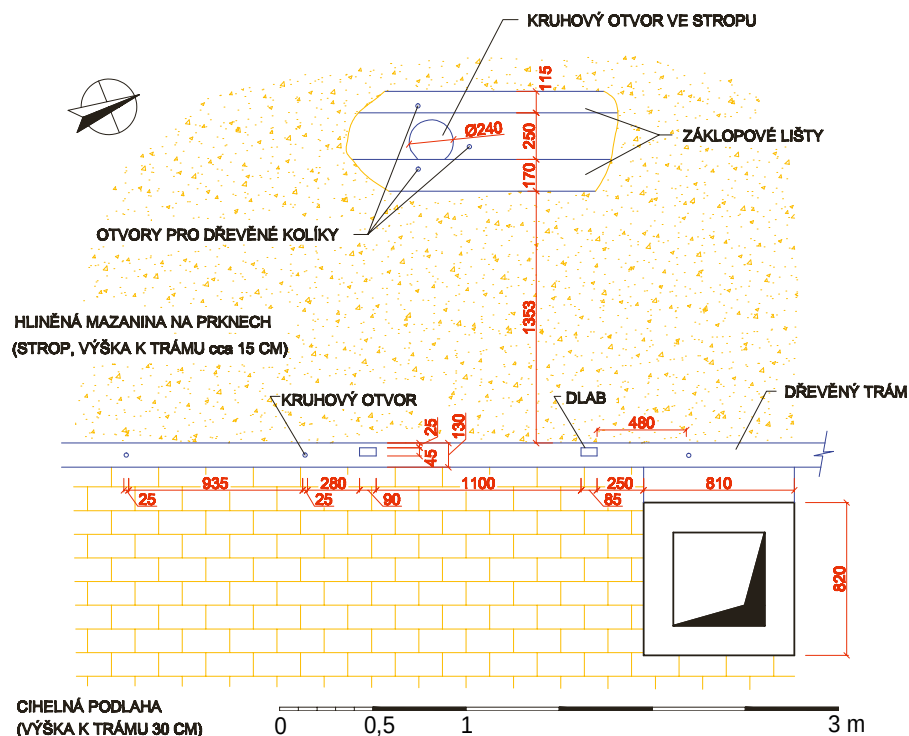
Obr. 16: Vyšší Brod, dům čp. 24, zákres rubové strany stropu světnice s vyříznutým kruhovým otvorem v záklopu a pozici dvou dlabů v posledním trámu roubení; kruhové otvory po kolících v tomto trámu jsou s nimi soudobé, sloužily patrně pro uchycení krokvi (zaměření a zákres V. Babická).
