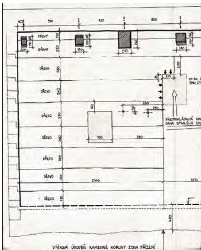
Obr. 48: Český Krumlov, Dlouhá čp. 90, roubená místnost v patře, zákres západní stěn se dvěma dochovanými okénky (zaměření a zákres F. Kápar).
