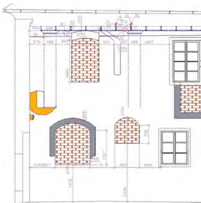
Obr. 55: Český Krumlov, Latrán čp. 67, hospodářský dvůr kláštera klarisek (zákres M. Špinarová).
