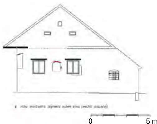
Obr. 36: Záluží – usedlost čp. 6, zákres průčelí obytného stavení s původní kompozicí třech oken.
