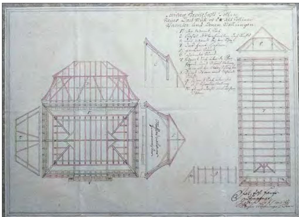
Obr. 7: Starý Kolín (okres Kolín), plán ke stavbě krovů nad farou a vedlejšími budovami od Matese Wolnera z roku 1764 (NA, APA I., kart. 1400).
