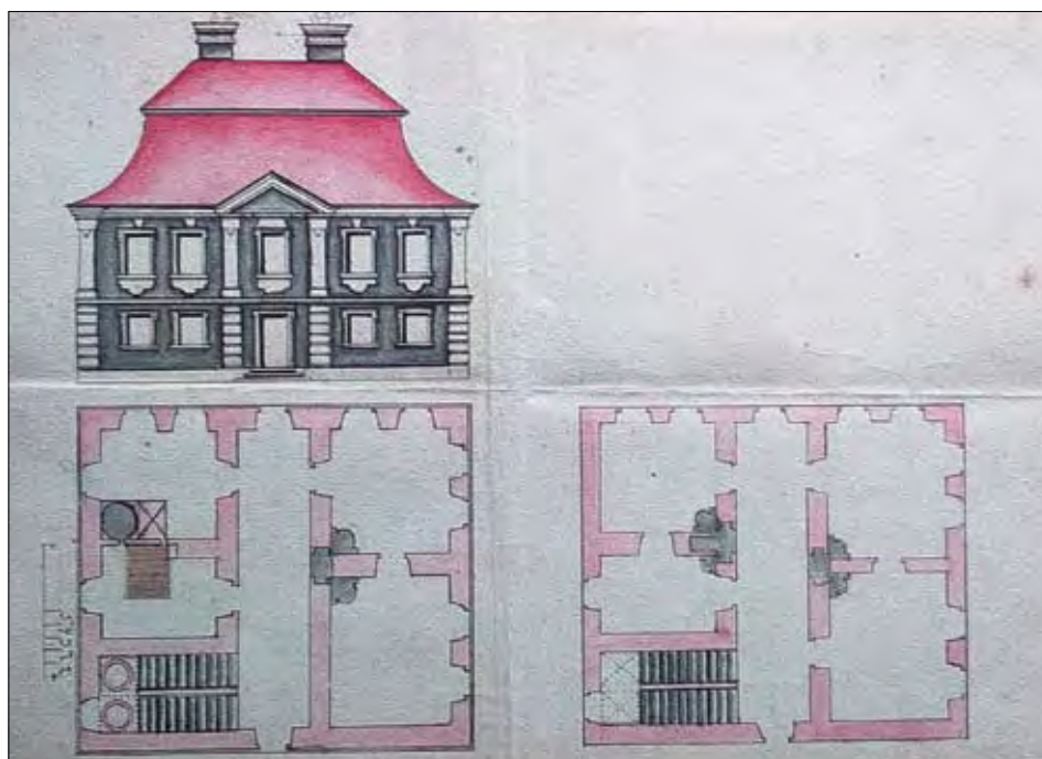
Obr. 12: Ronov nad Doubravou (okres Chrudim), plán ke stavbě fary od Josefa Jedličky z r. 1747 (NA, APA I., kart. 1301).
