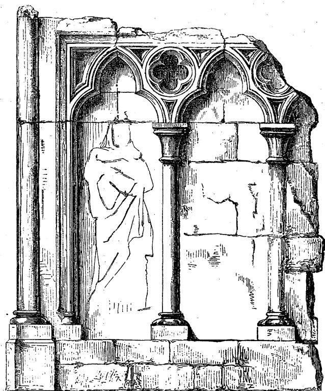
Obr. 4: Hrad v Písku, sedile v hradní kapli podle B. Gruebera.
